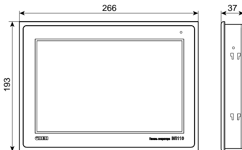
Рисунок 4.1 – Габаритные размеры
